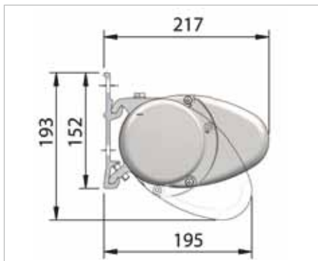
BRUSTOR B-50 avec fixation murale
