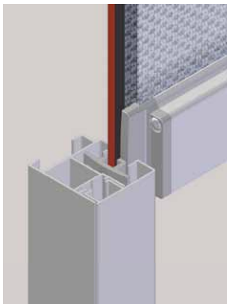
Le screen résiste au vent grâce à l'ingénieux système de fermeture éclair.
