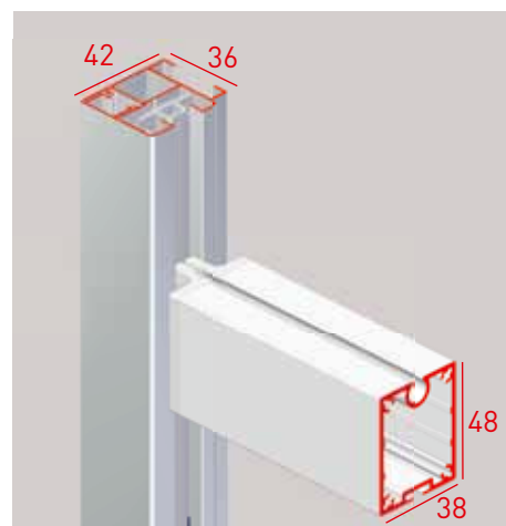
Glissière pour B-1350 C ZIP.
