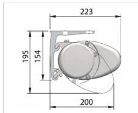
BRUSTOR B-50 avec fixation plafond (sans plus-value)
