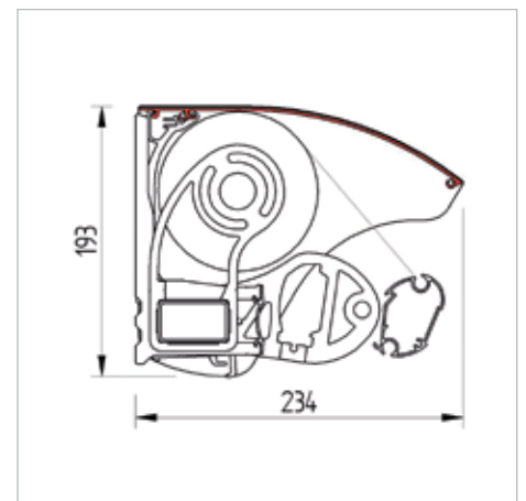
B34 AVEC AUVENT
