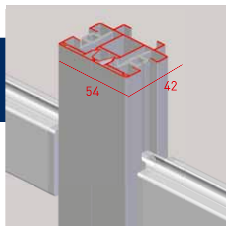
Glissière pour B-1085 ZIP couplé et B-1100 ZIP couplé.
