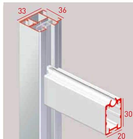
Glissière pour B-1085 ZIP et B-1100 ZIP.
