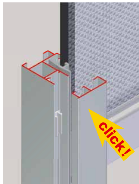
Le screen Zip possède des coulisses uniques qui se ferment en les cliquant lors du montage. Les trous de perçage ne sont pas visibles.
