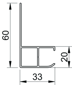
en option: glissière side fix 60mm P x 33mm L
