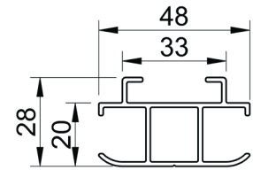
glissière couplée 28mm P x 48mm L
