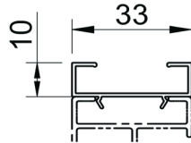
en option: cale de rattrapage 10mm P x 33mm L
