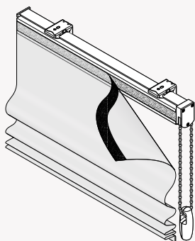
Type C : Manœuvre chaînette relevage cordon
